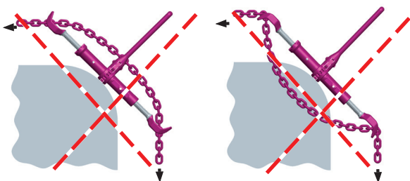
Bild 13: Verbotene Biegebelastung
