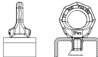
Abb. 1: Blindnietmutter
