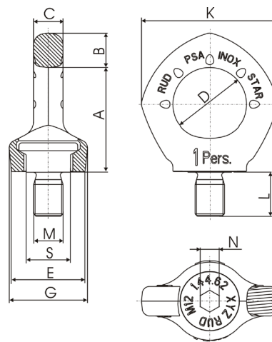
Maßzeichnung PSA INOX STAR
