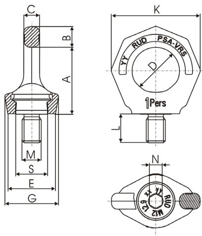
Maßzeichnung PSA-VRS
