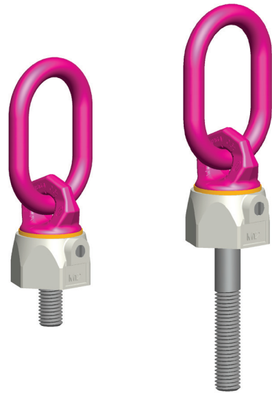
Wirbelbock-Gewinde (Vario) VWBG-V
