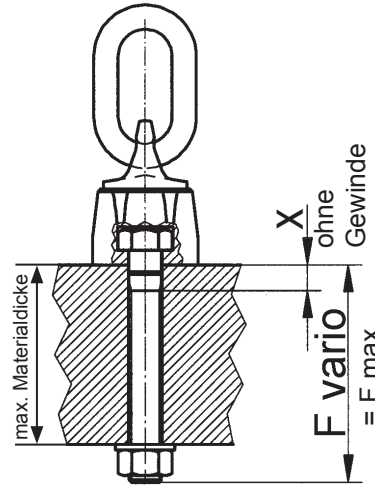
Abb. 4: Bemaßung VWBG-V
