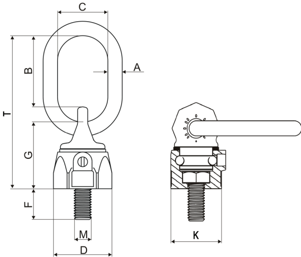
Abb. 3: Bemaßung VWBG-V
